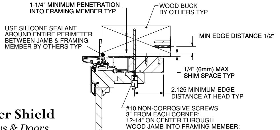
SECTION B-B SCALE 1 : 4
